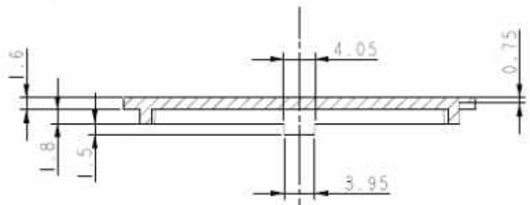
Ausschnitt A-A
