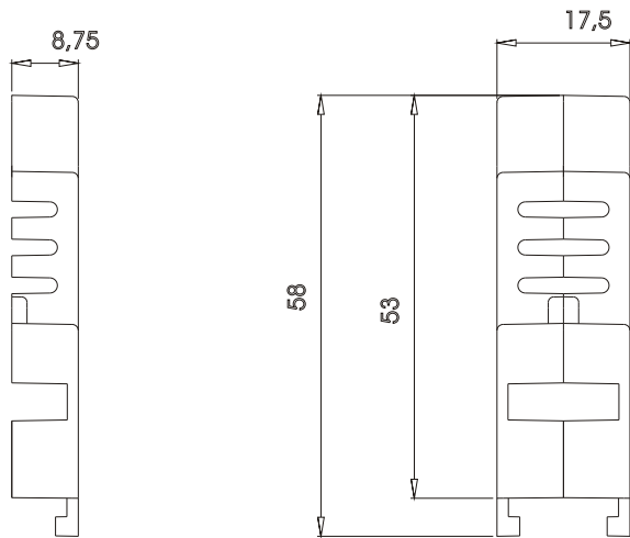
Leiterplattenmaße
