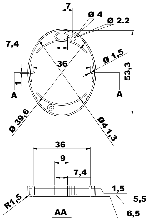
Unterteil
